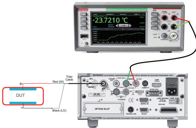
信号连接图
