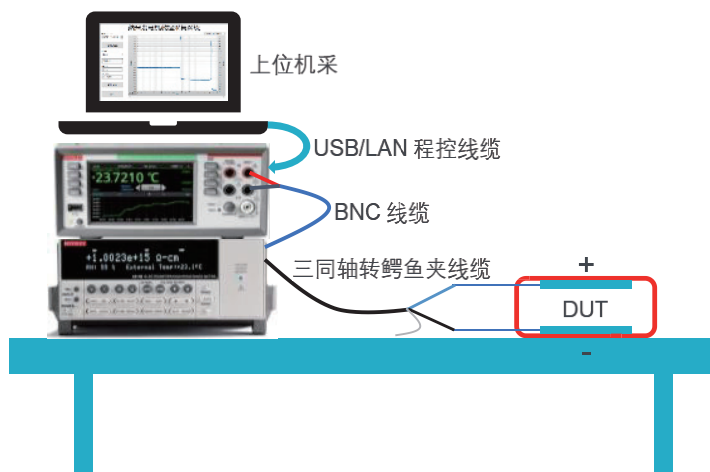
配置图
